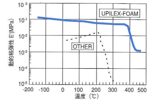
図2 ユーピレックス フォームの動的粘弾性線(室素中)
