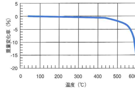
図1 ユーピレックス フォームの熱重量減少曲線(空气中)
